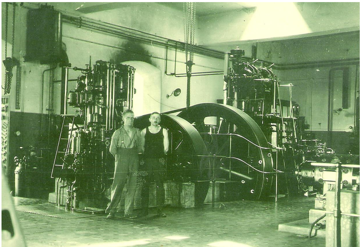
Dieselmotoren des Elektrizitätswerkes Waidhofen um 1920
